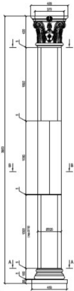
Колонна Коринфский ордер D=320 KL.320K
